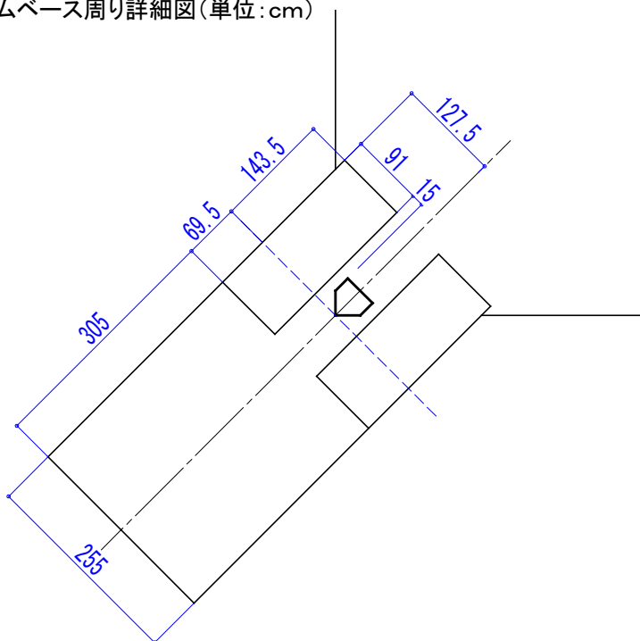
ホームベース周り詳細図(単位:cm)
